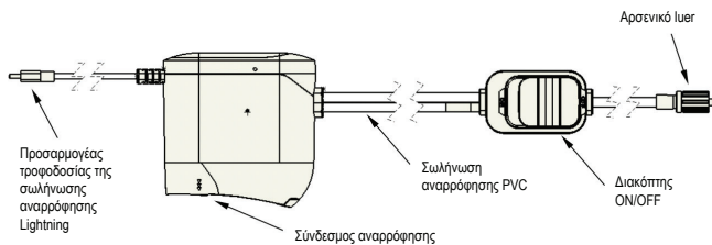
Εικόνα 2: Σωλήνωση αναρρόφησης Lightning
