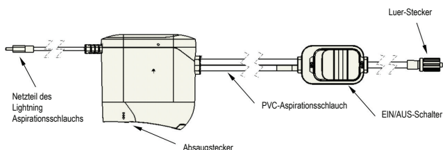
Abbildung 2: Lightning Aspirationsschlauch
