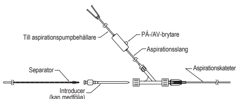
Figur 1: Monterad Lightning Aspirationsslang med INDIGO Aspirationssystem
