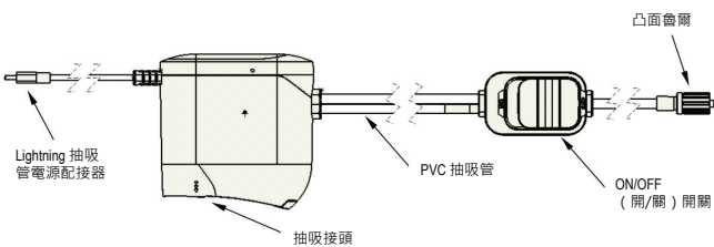
圖 2：Lightning 抽吸管
