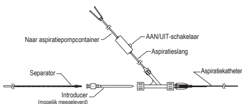
Afbeelding 1: Opgebouwde Lightning-aspiratieslang met INDIGO-aspiratiesysteem
