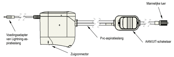
Afbeelding 2: Lightning-aspiratieslang
