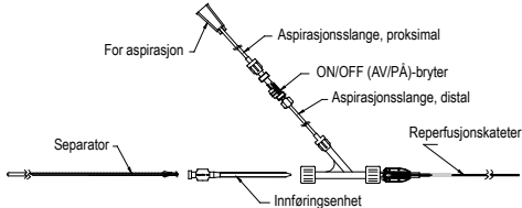
Figur 1 – Montert aspirasjonssystem med Penumbra Separator
