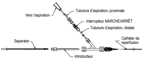
Figure 1 – Système d'aspiration assemblé avec le Penumbra Separator
