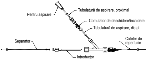
Figura 1 – Sistemul de aspirare asamblat cu Penumbra Separator
