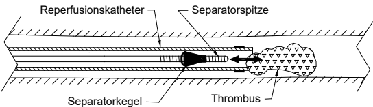
Abbildung 2 – Thrombus-Aspiration mithilfe des Penumbra Separators
