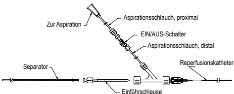
Abbildung 1 – Montiertes Aspirationssystem mit Penumbra Separator
