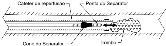
Figura 2 — Aspiração do trombo utilizando o Penumbra Separator
