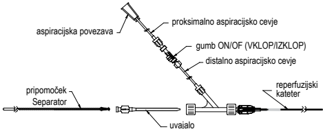
Slika 1 – aspiracijski sistem z nastavljenim pripomočkom Penumbra Separator
