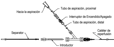
Figura 1. Sistema de aspiración ensamblado con Separator de Penumbra
