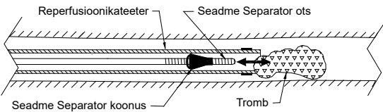
Joonis 2 – trombi aspireerimine seadmega Penumbra Separator
