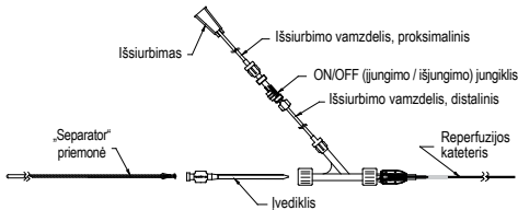
1 pav. Surinkta išsiurbimo sistema su „Penumbra Separator“
