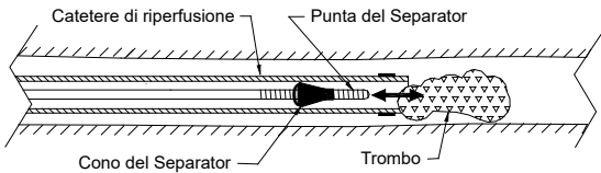
Figura 2 – Aspirazione del trombo tramite il Separator Penumbra
