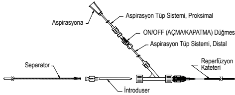
Şekil 1 – Penumbra Separator İçeren Monte Edilmiş Aspirasyon Sistemi
