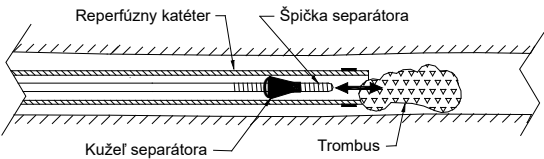
Obrázok 2 – Aspirácia trombu pomocou Penumbra Separator
