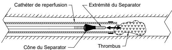
Figure 2 – Aspiration d'un thrombus à l'aide du Penumbra Separator
