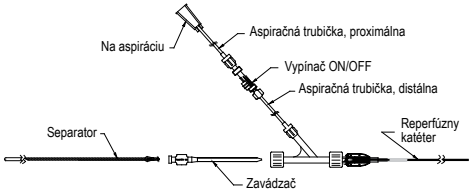
Obrázok 1 – Zmontovaný aspiračný systém so separátorom Penumbra Separator
