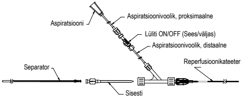
Joonis 1 – kokkupandud aspiratsioonisüsteem koos seadmega Penumbra Separator
