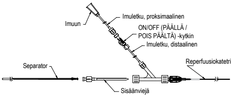
Kuva 1 – Koottu imujärjestelmä ja Penumbra Separator -laite
