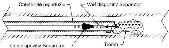
Figura 2 - Aspirarea trombului cu ajutorul dispozitivului Penumbra Separator
