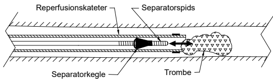
Figur 2 – Trombeaspiration med Penumbra-separatoren
