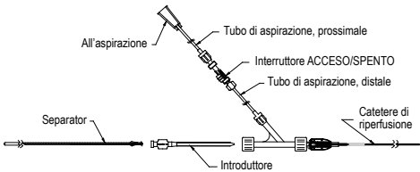
Figura 1 – Sistema di aspirazione montato con il Separator Penumbra
