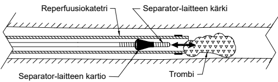
Kuva 2 – Trombin aspirointi Penumbra Separator -laitteella
