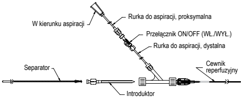
Rysunek 1 – Złożony system aspiracji wraz z separatorem Penumbra
